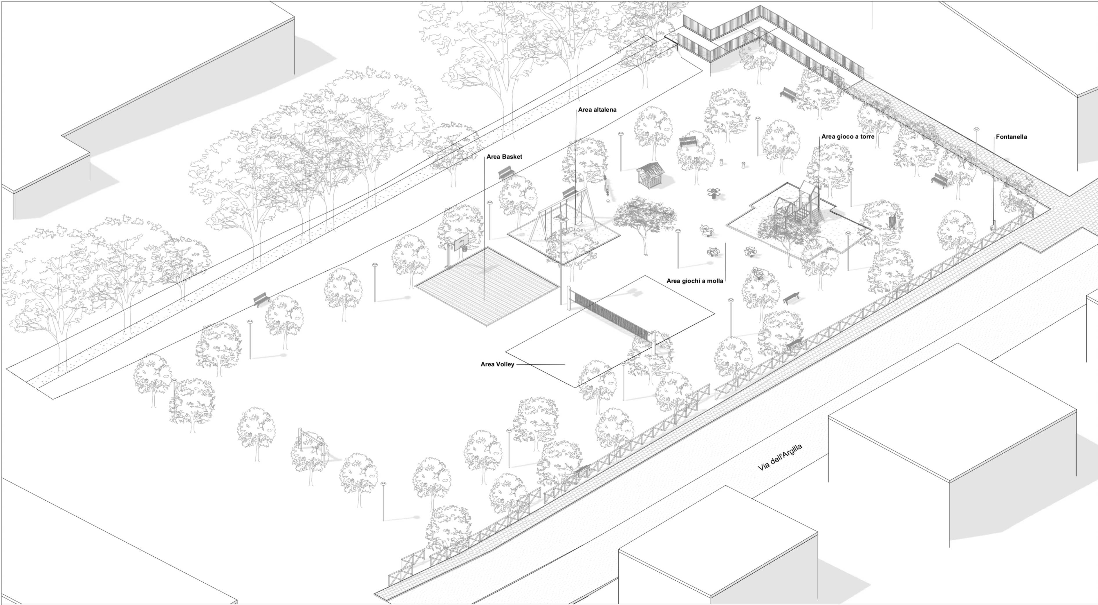
VISTA ASSONOMETRICA DELLO STATO ATTUALE SCALA 1:200
