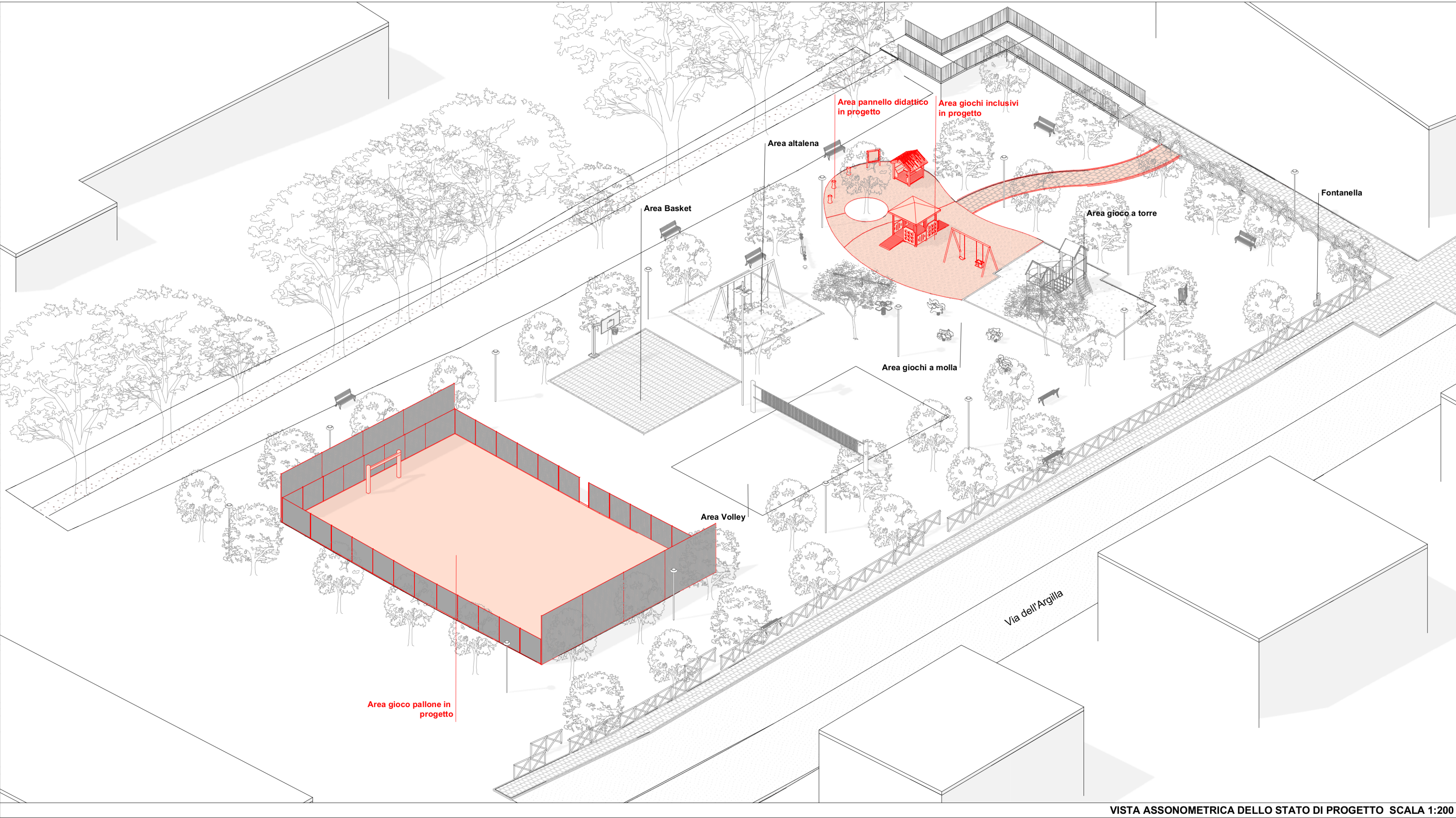
VISTA ASSONOMETRICA DELLO STATO DI PROGETTO SCALA 1:200
