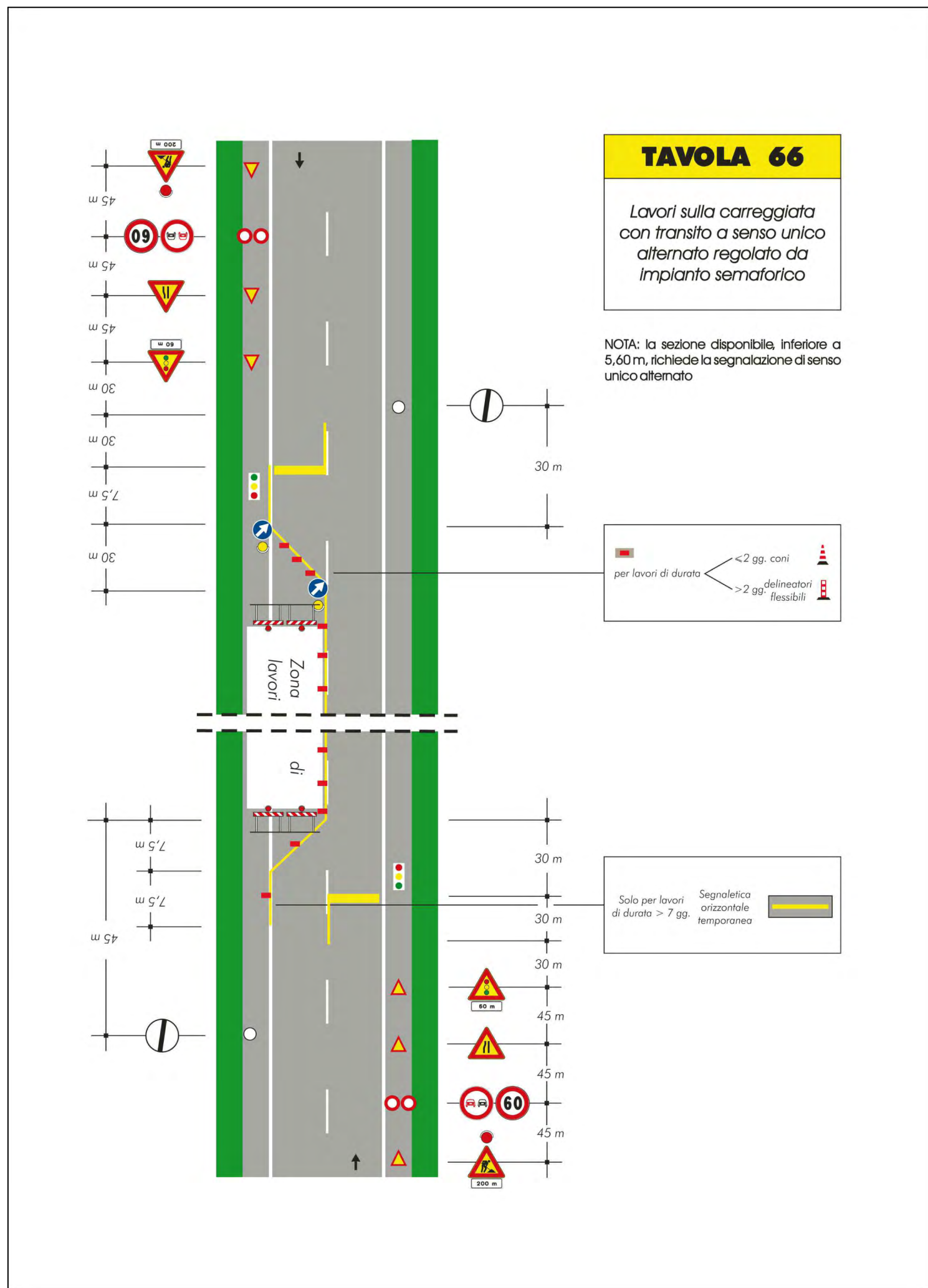
IMM. 4 POSIZIONAMENTO IMPIANTO SEMAFORICO - D SOTTOCANTIERE 2
