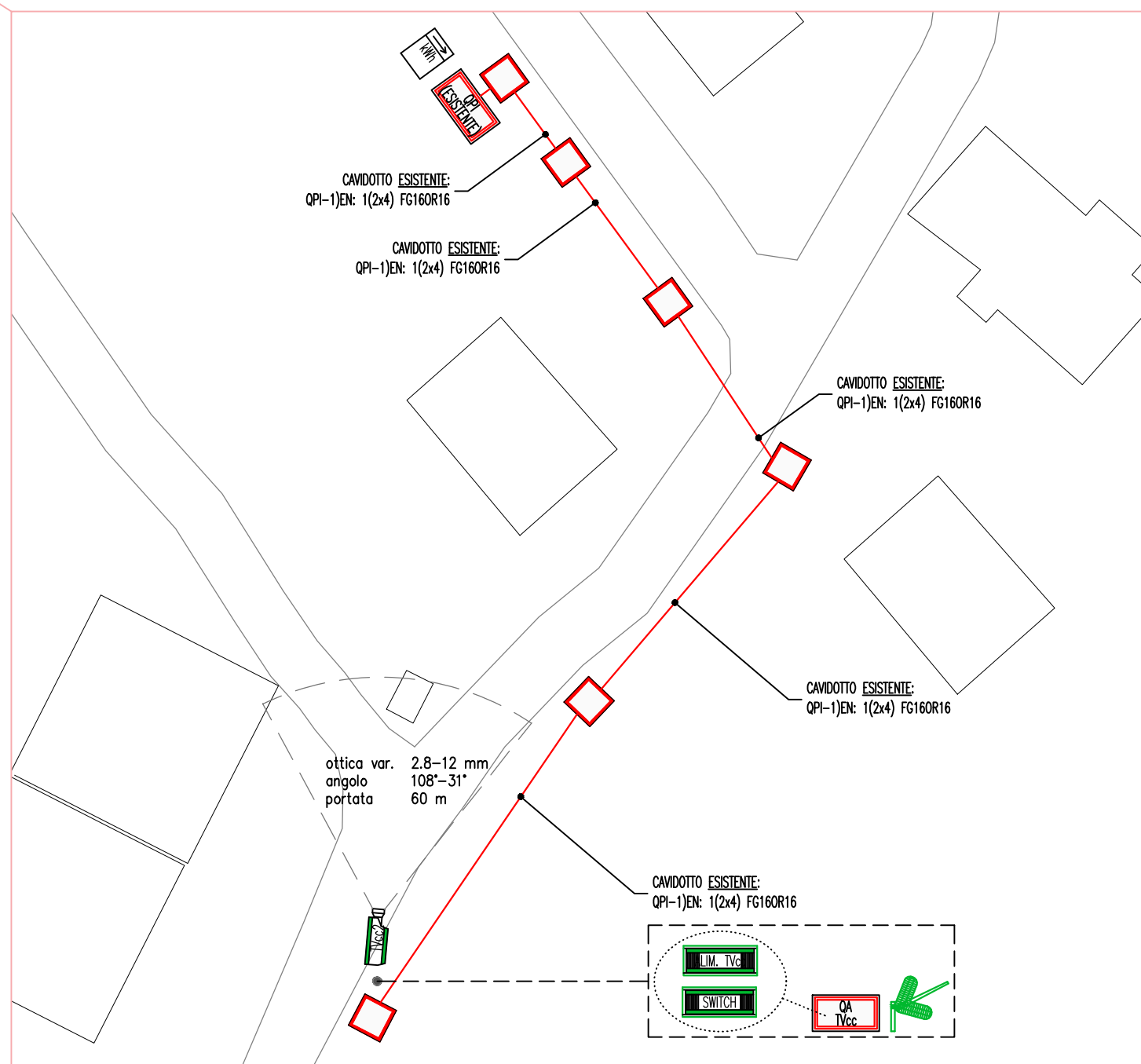
CASTELLEONE scala 1:500
