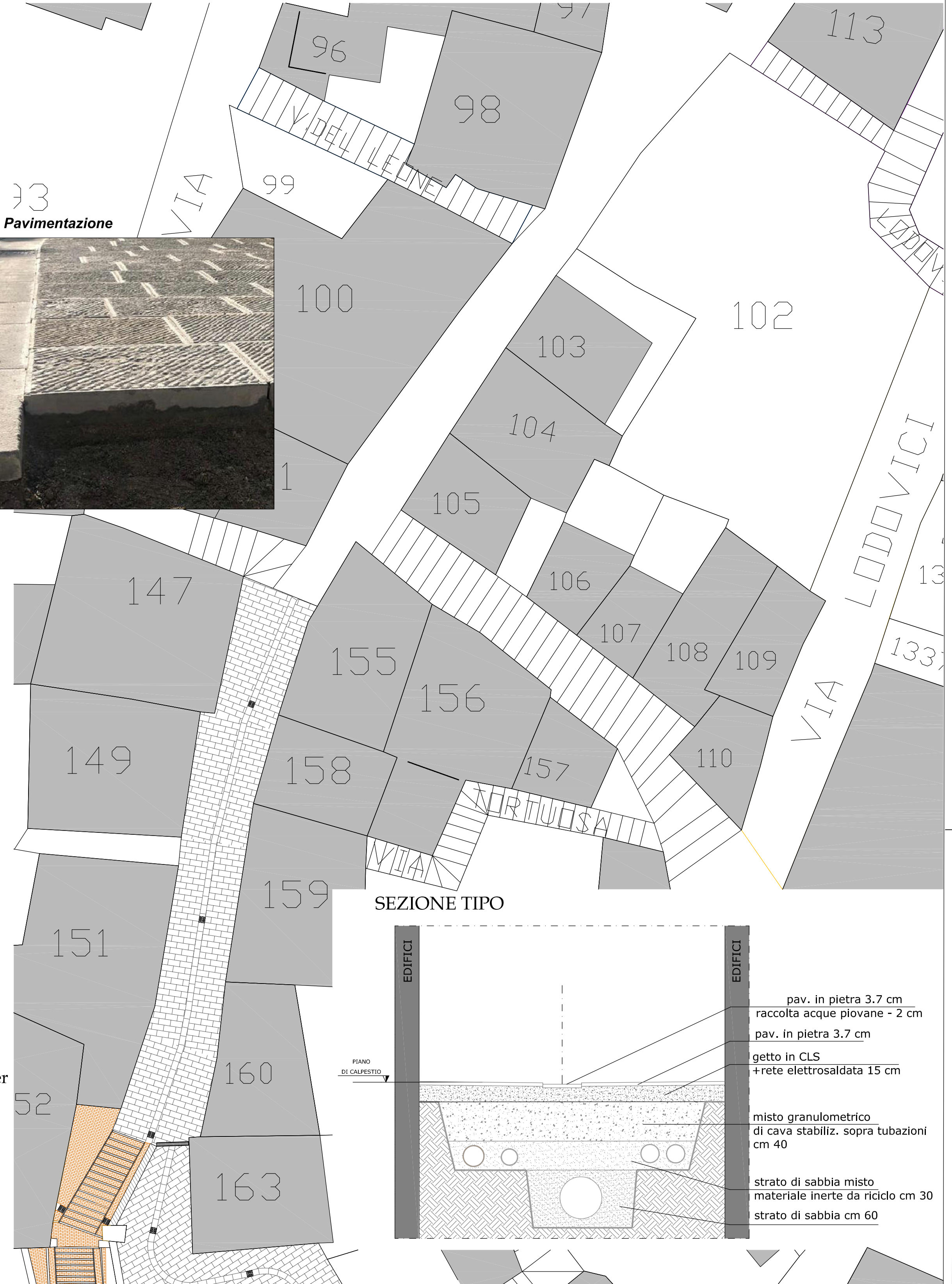
VIA MATURANZIO 1° TRATTO - SCALA 1:200
