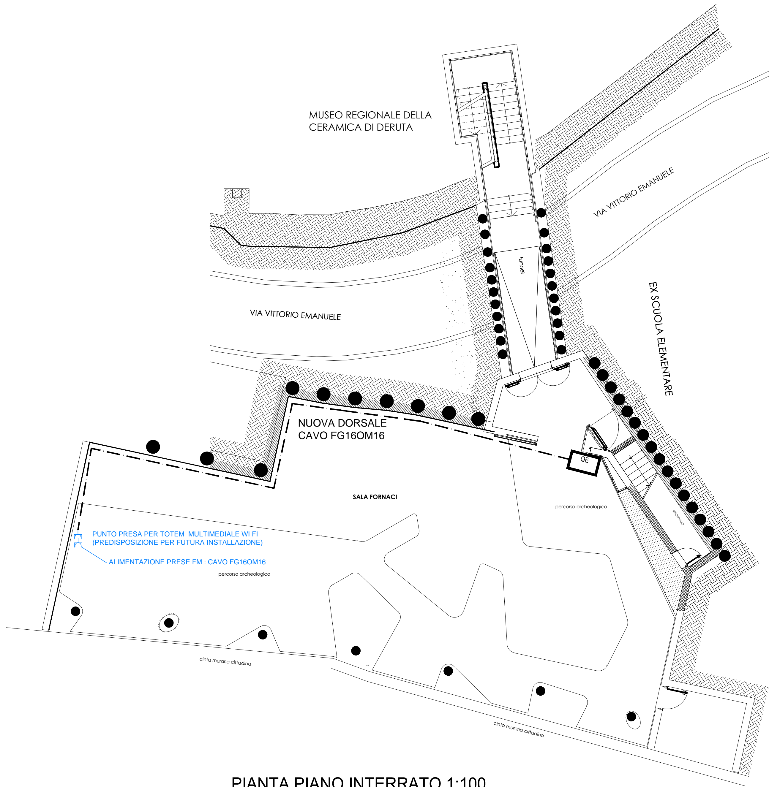
PIANTA PIANO INTERRATO 1:100
